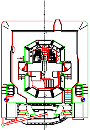
Bridgedeck
